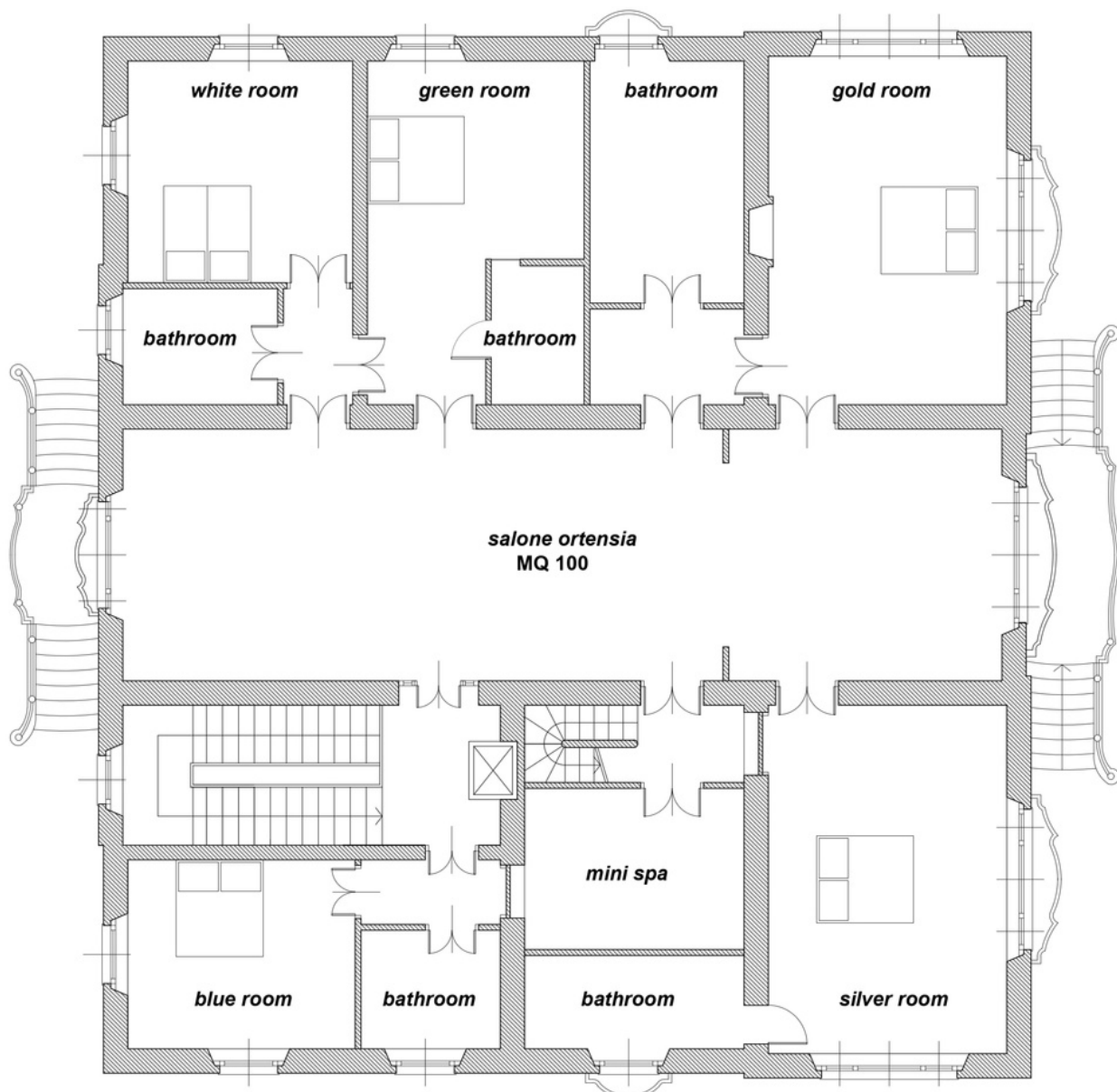
pianta piano primo | first floor map
